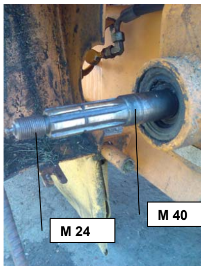
Hriadeľ pohonu k ŽTR 330 na ktorú sa nasadzuje zubová spojka
