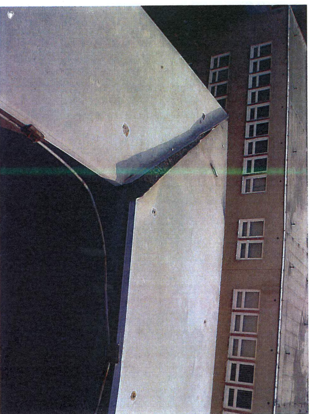
Poškodené, uvoľnené oplechovanie atíky, ktoré drží uzemňovací vodič
