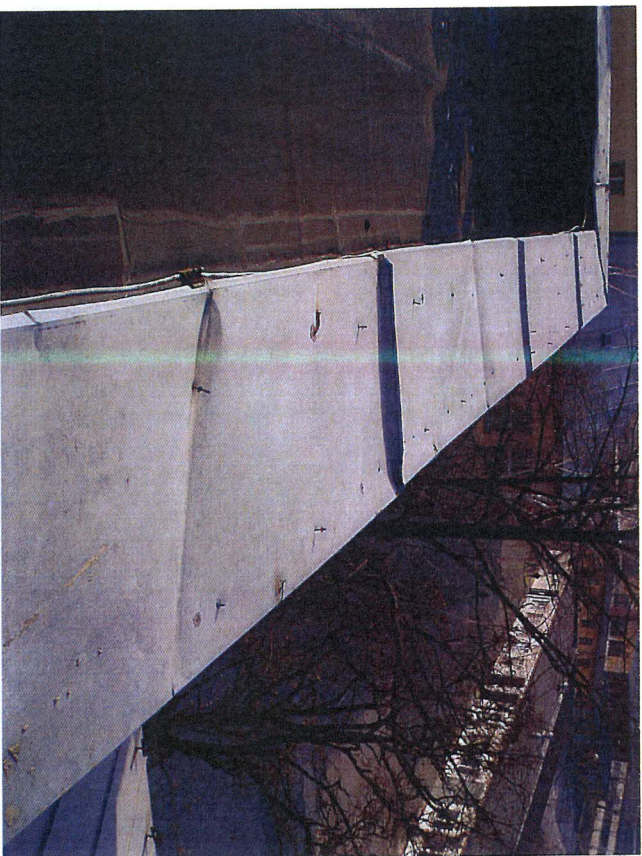
Detailný pohľad na uvoľnené upevňovacie klince
