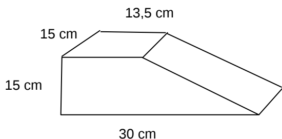
Obr. 1: Klin drevený
