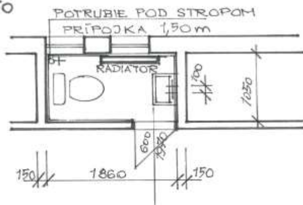
PÔDORYS M 1:50
