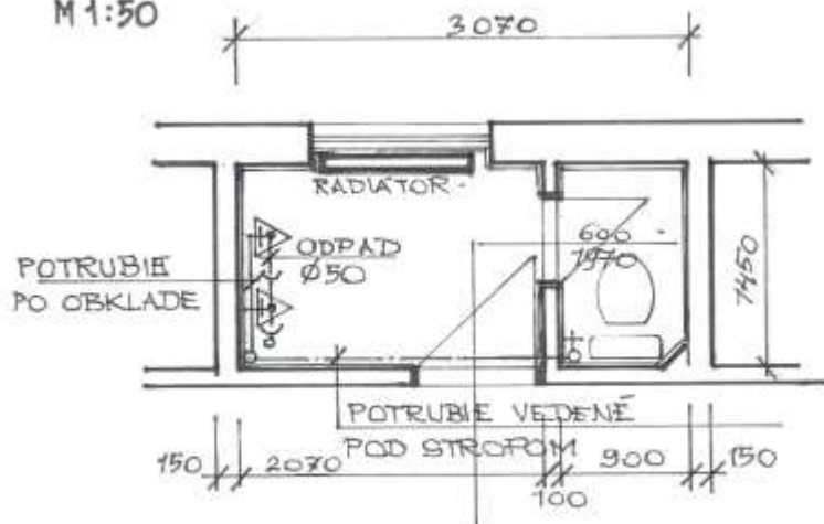
PÔDORYS M 1:50
