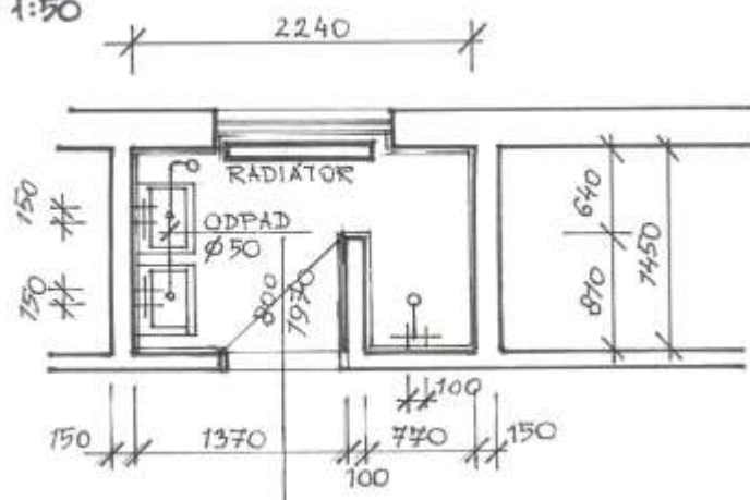
PÔDORYS M 1:50
