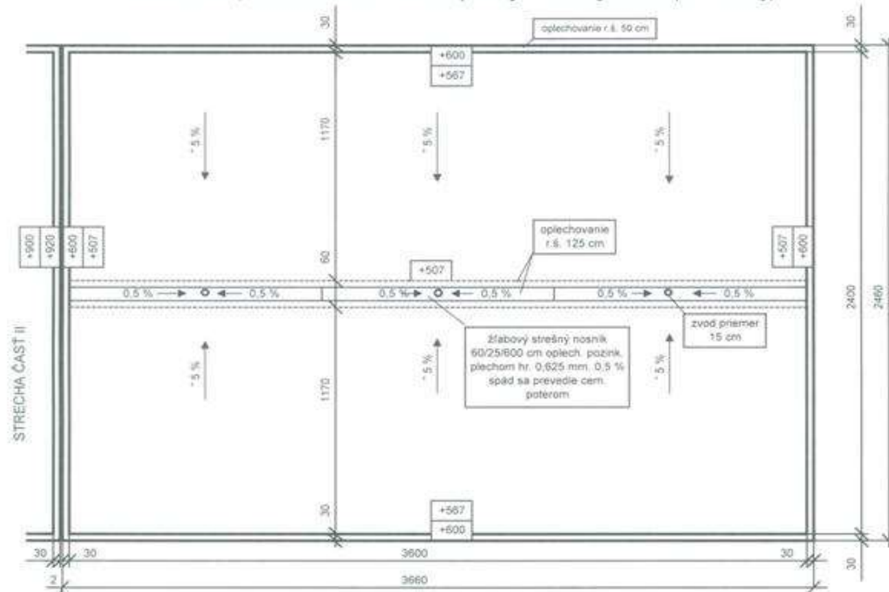
K SNP Martin, Budova číslo 97 - Náčres pôdorysu strechy časť III (bez mierky)
