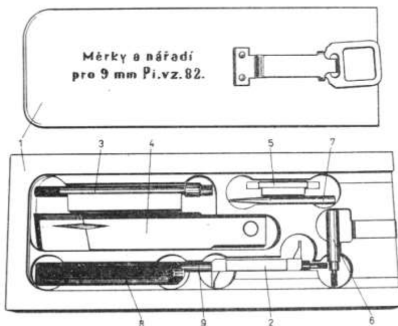
Súprava mierok a náradia pre Pi vz. 82
